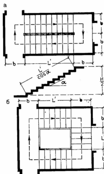
Рис. П5.1. Расчетная длина пути по лестнице: а - двухмаршевая лестница; б - трехмаршевая лестница
