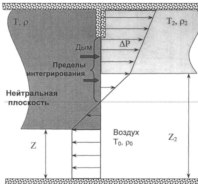
Рис. Пб.1. Массопотоки через проем
