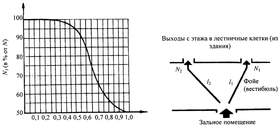
Рис. П5.5, а. Число зрителей и выбор выхода при эвакуации в две лестничные клетки либо в две открытые лестницы или в два выхода из здания:
