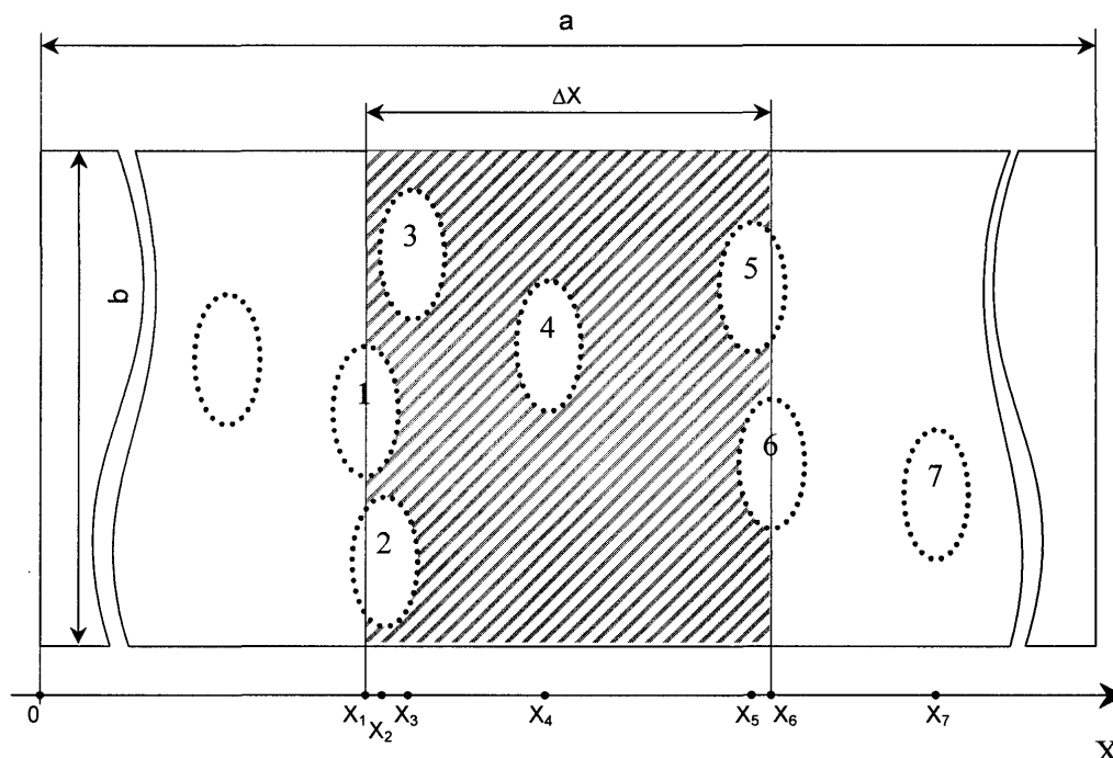
Рис. П3.1. Координатная схема размещения людей на путях эвакуации
