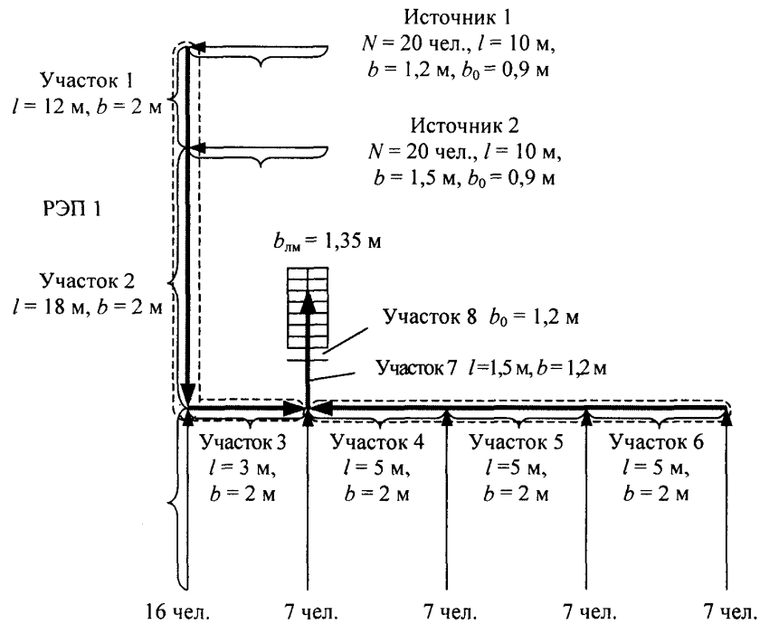
Рис. П5.2. Пример составления расчетной схемы эвакуации людей по части этажа до входа в лестничную клетку:
